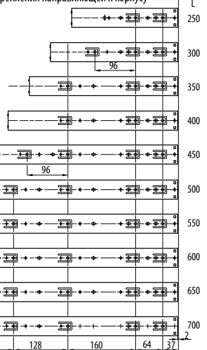
Место крепления направляющей к корпусу
