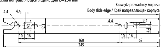
Схема направляющей ящика для L=250 мм
