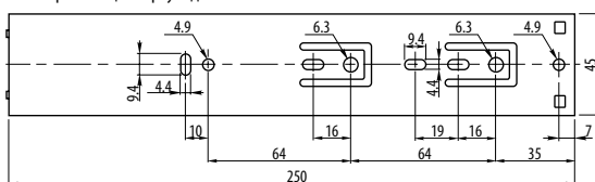
Схема направляющей корпуса для L=250 мм
