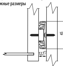
Pozycja mocowania prowadnic korpusu Fixing position of body slides
